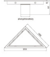
HY-DL66 Floor drain ตะแกรงกันกลิ่น ฿585
